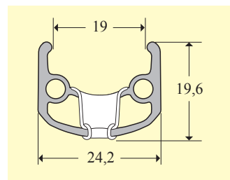
EXAL Felge SP19
