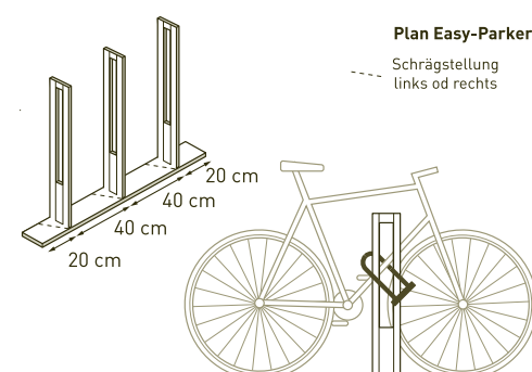
HE- mit Bodenstütze und Quertraverse
